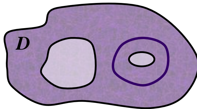
复连通区域
